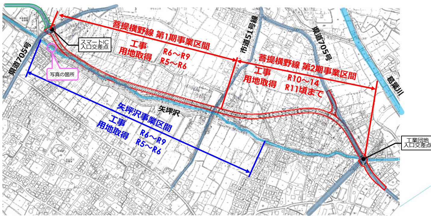
菩提横野線街路整備事業 延長1280m 道路幅16m
