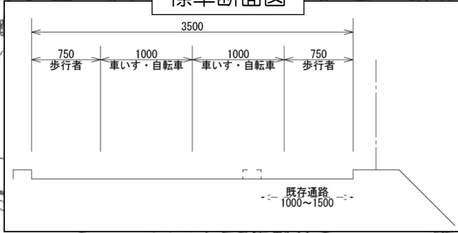
標準断面図
