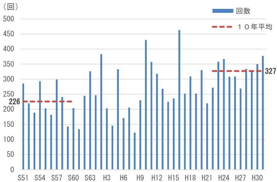
図表 2-1 全国の 1 時間降水量 50mm 以上の年間発生回数
