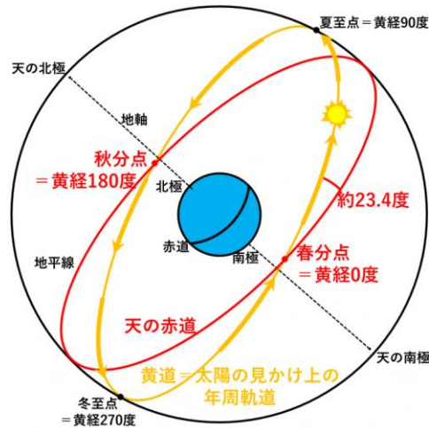
太陽の年周軌道における春分点と秋分点の位置
