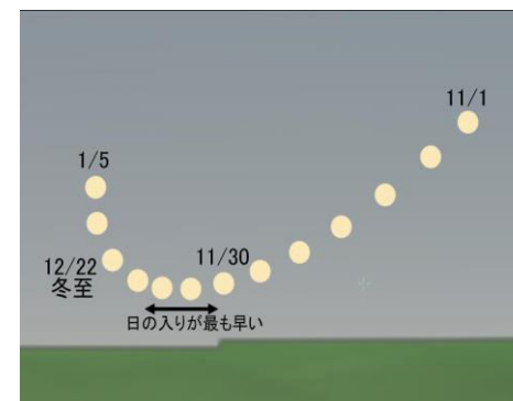
冬至前後、西の空 16 時の太陽の位置
