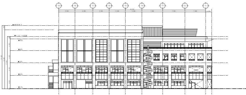
觀景北側立面圖
