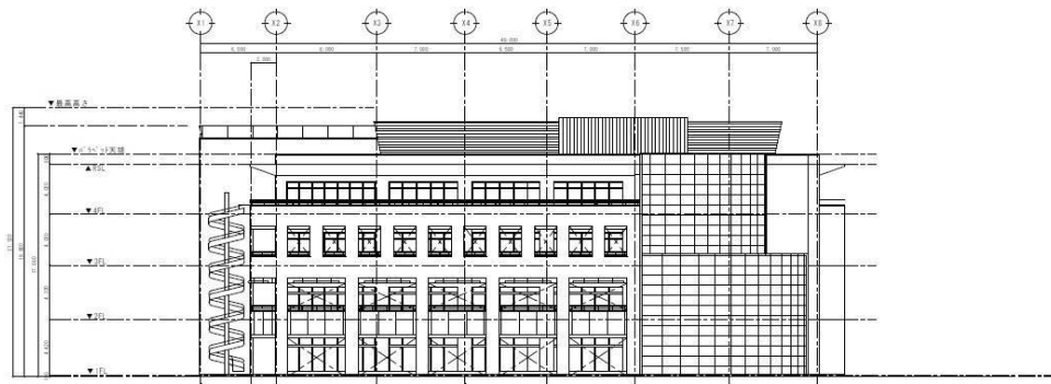
觀景西側立面圖
