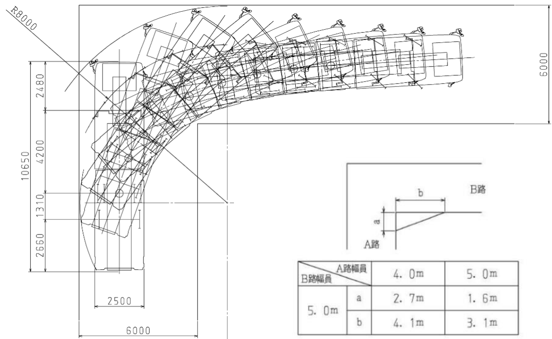
はしご車走行に係る道路等隅切り表
