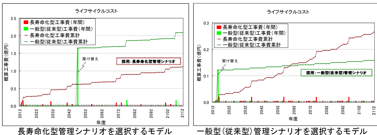
図-4.1 長寿命化型管理と一般型(従来型)管理のライフサイクルコスト比較
