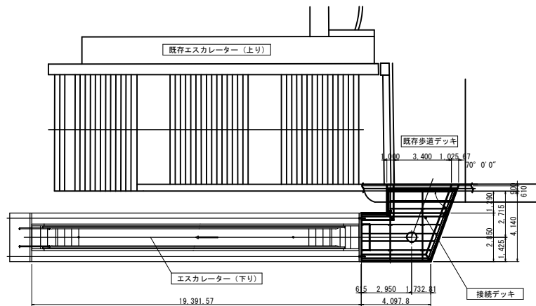
平面図
