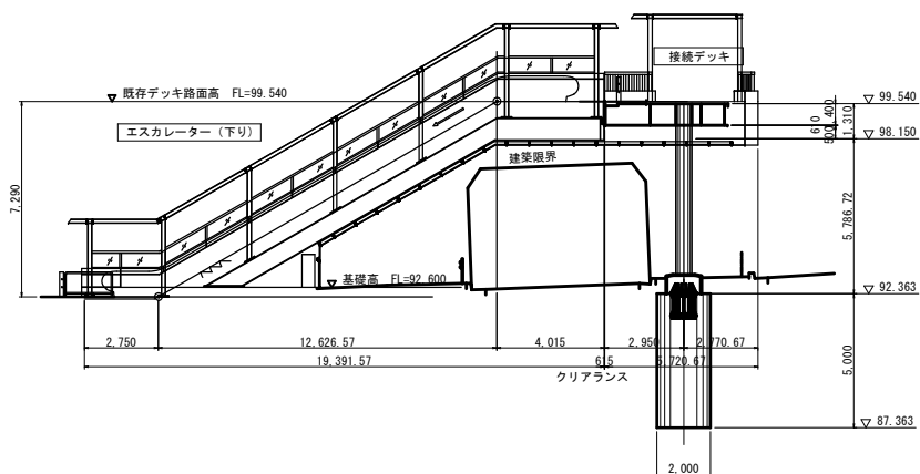
側面図
